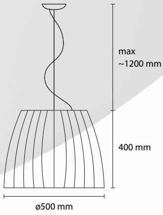
SP SOL 50 3 E27 42W ALO
