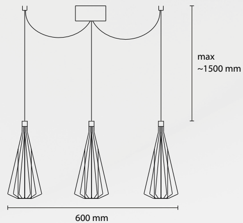
SP GHIAC 3 / 18 3 E14 28W ALO
