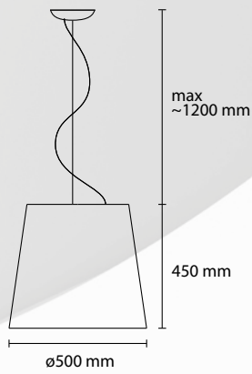
SP ROSE 50 1 E27 54W
