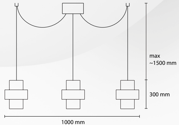
SP OLIMPO 3 / 24 3 E14 28W ALO
