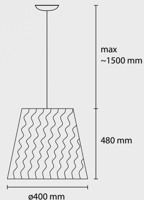
SP STOK 40 1 E27 42W ALO
