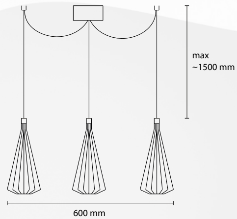
SP ECO 3 / 18 3 E14 28W ALO
