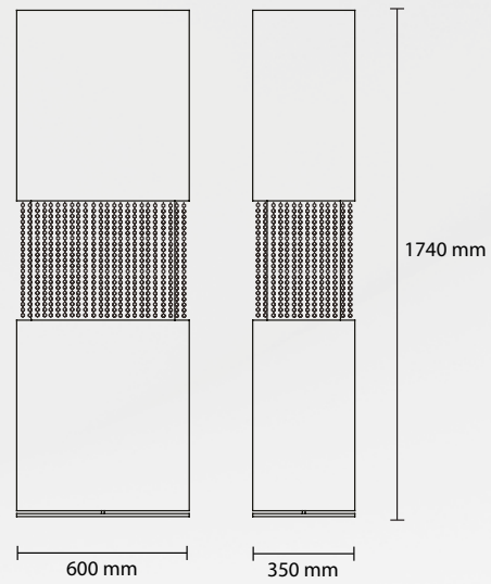
PT CRISTAL Q 174 4 E27 42W ALO
