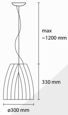
SP SOL 30 1 E27 35W ALO
