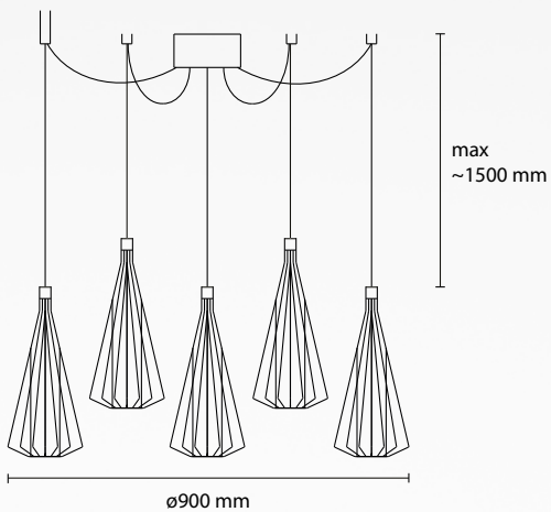
SP GHIAC 5 / 18 5 E14 28W ALO
