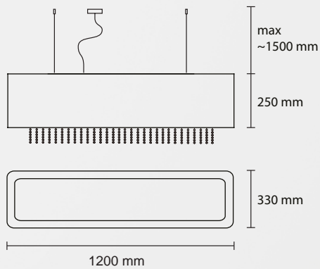
SP CRISTAL Q 120 4 E27 42W ALO
