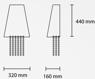
AP BOLLO 32 1 E27 42W ALO
