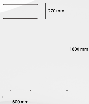
PT BUGHY 180 3 E27 42W ALO
