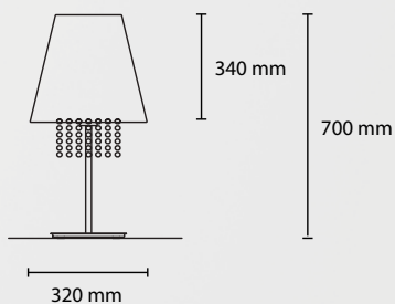
LT BROLLO 70 1 E27 42W ALO
