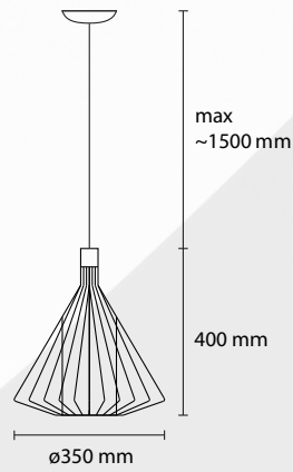
SP GHIAC 35 1 E27 42W ALO
